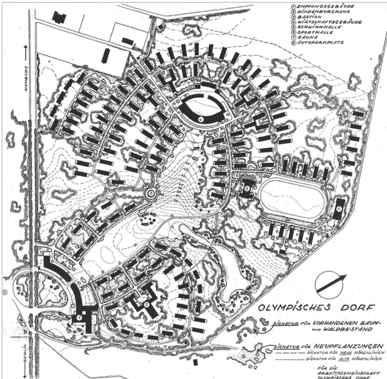
Abb. 2: Lageplan von 1936; Wiepking-Jürgensmann 1936
