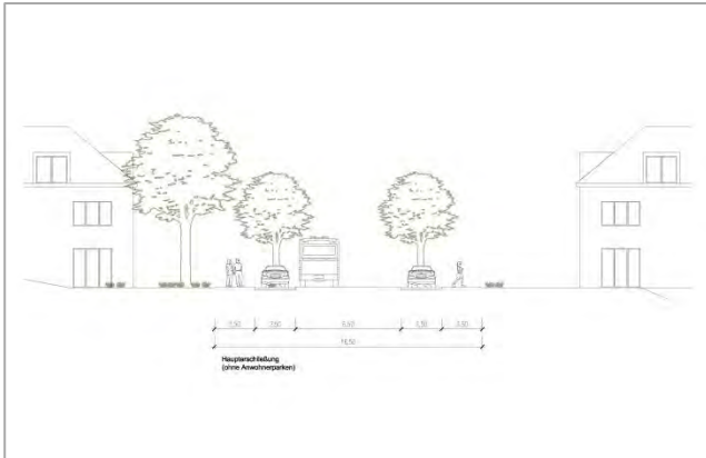
Abb. 39: Straßenschnitt öffentliche Haupteinschließung mit öffentlichen Stellplätzen
