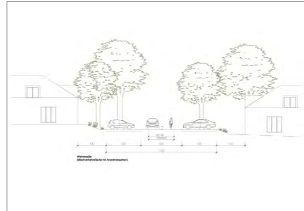
Abb. 40: Straßenschnitt Wohnstraße mit privaten Stellplätzen
